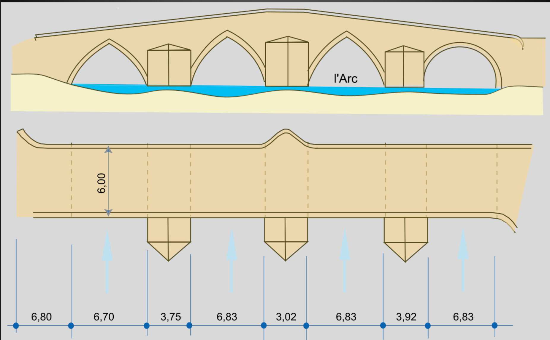
PLAN DU PONT DE SAINT-PONS
